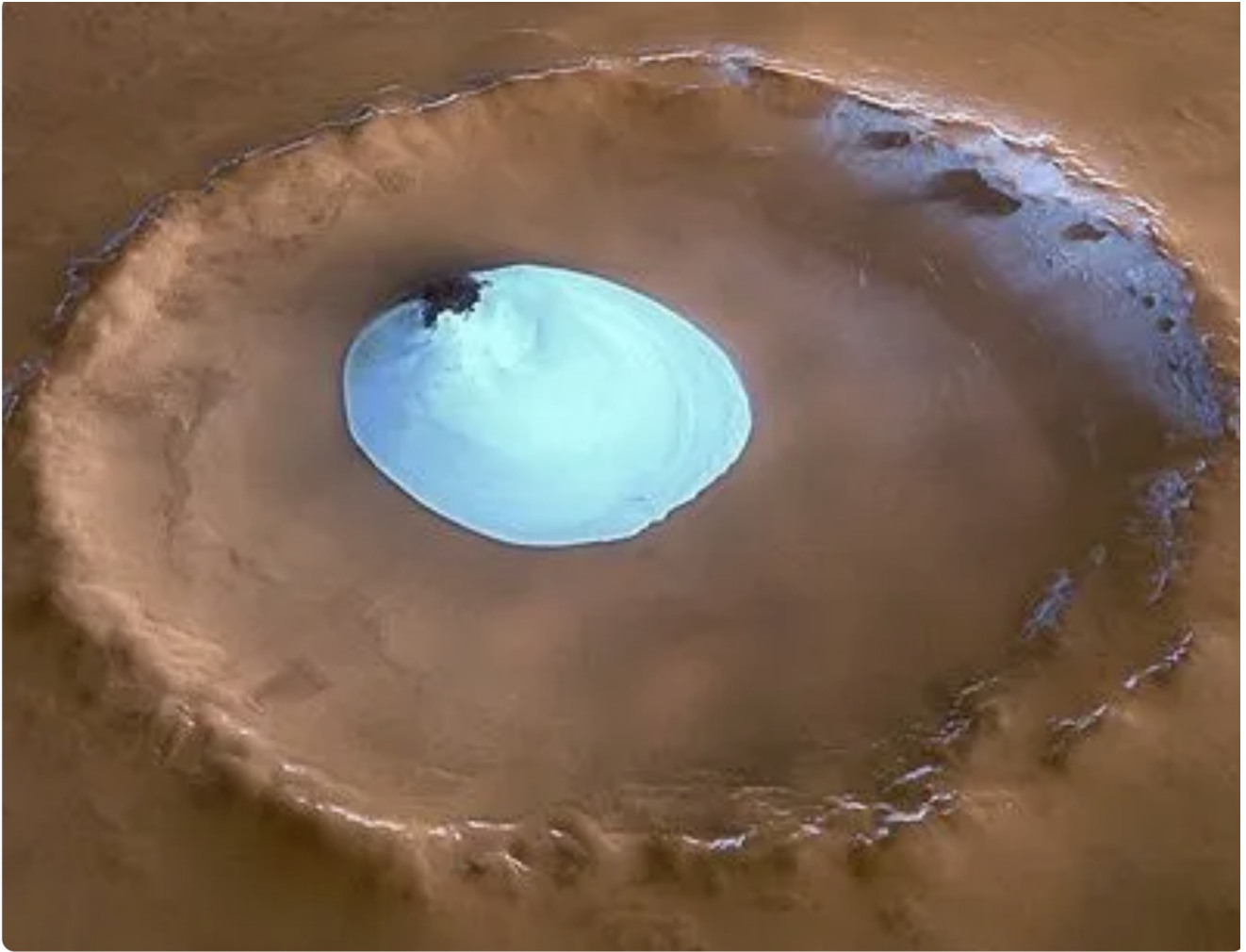
Mars: eau glacée dans un cratère du pôle nord
