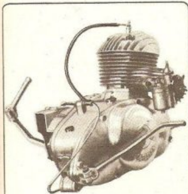
Bloc-moteur "Ydral" 2 temps, 125 cm 3 Vitesse en palier : 75 km. à l'heure. Consommation : 2 litres 3/4 aux 100 km.
