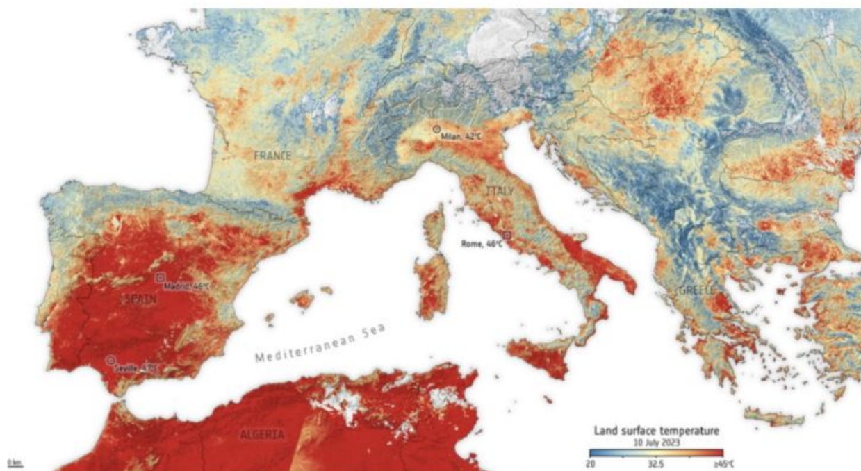
Diagramme de température de surface : Agence spatiale européenne (ESA)
